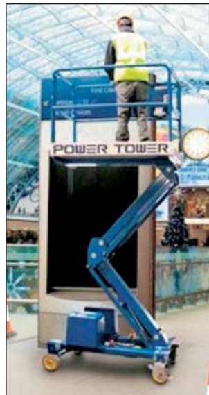
Piattaforma di lavoro mobile elevabile verticale (A1)
