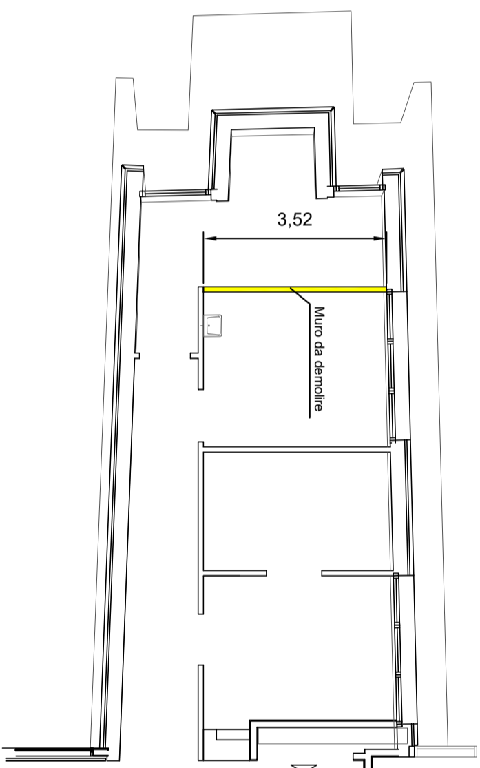
Raffronto Piano 7 - uffici coordinatrice pediatria H = 3.00 mt
